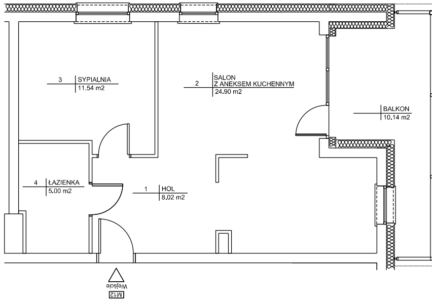
RZUT LOKALU
