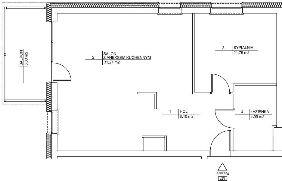
RZUT LOKALU
